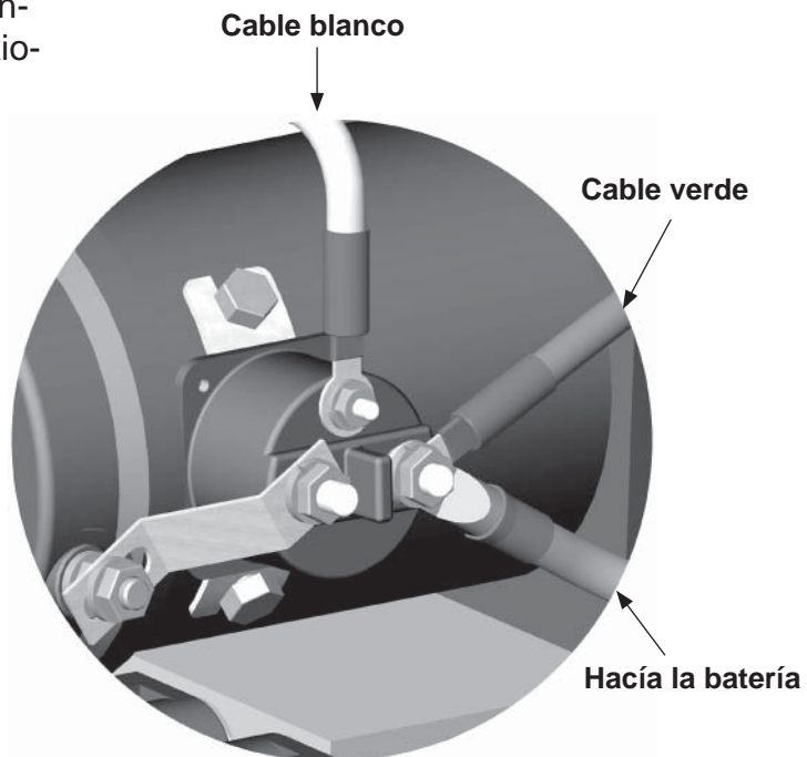
Solenoide del motor actual Fig. 32-2
