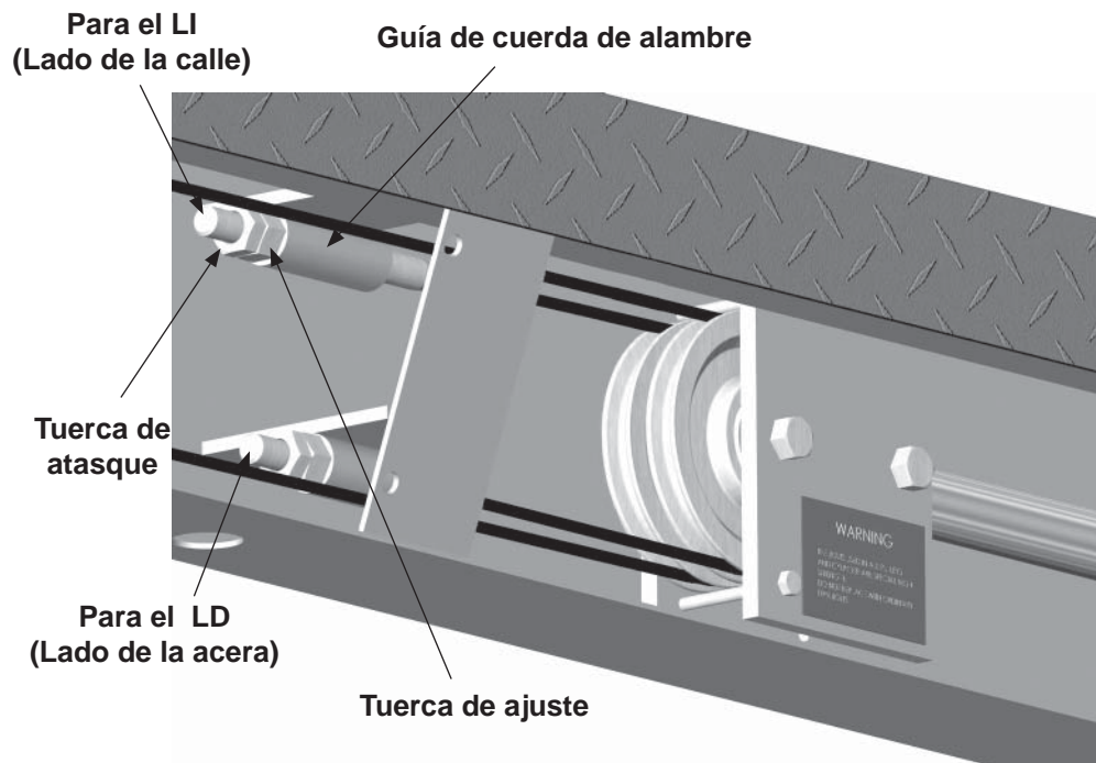
Ajuste de cuerda de alambre LI Fig. 40-1
